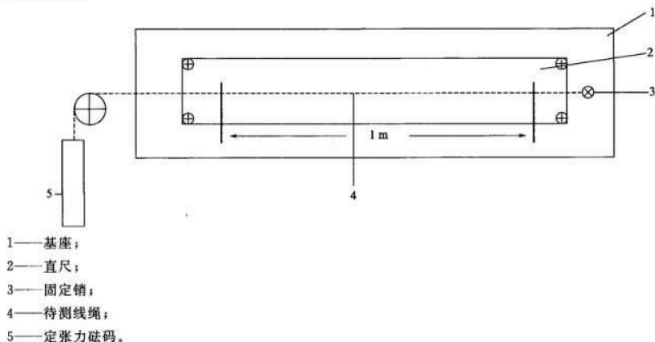
图 B.1 定张力制样器示意图
